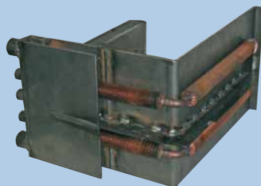
Schnittdarstellung mit innenliegender Kupferspirale
