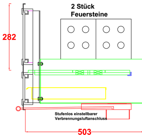
TZ: BRS Seitenansicht
