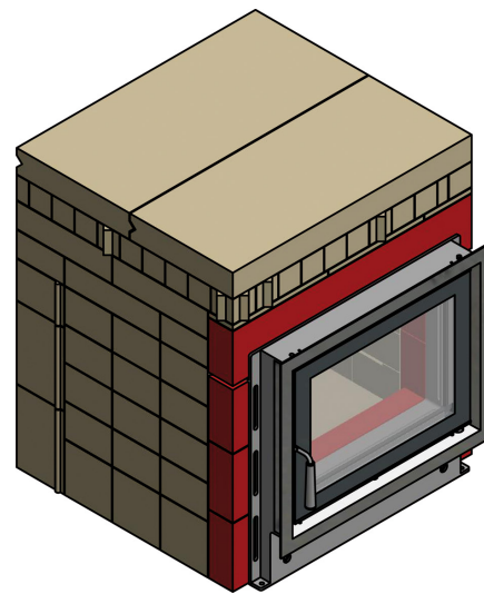
Grundofen-Brennraum
