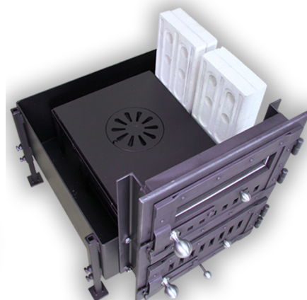
BRS Seitenansicht mit Platte & Feuerrost
