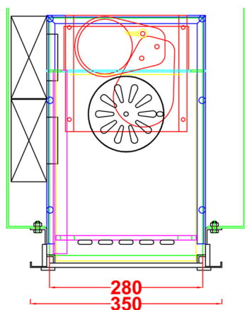
TZ: BRS Draufsicht mit Feuerrost
