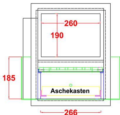
TZ: Frontansicht Rahmen ohne Türen
