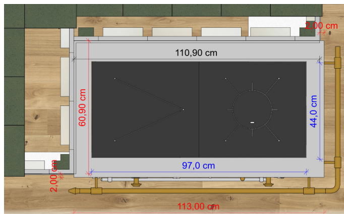
Planungsskizze mit Palette CAD: Herdrahmen und Platte
