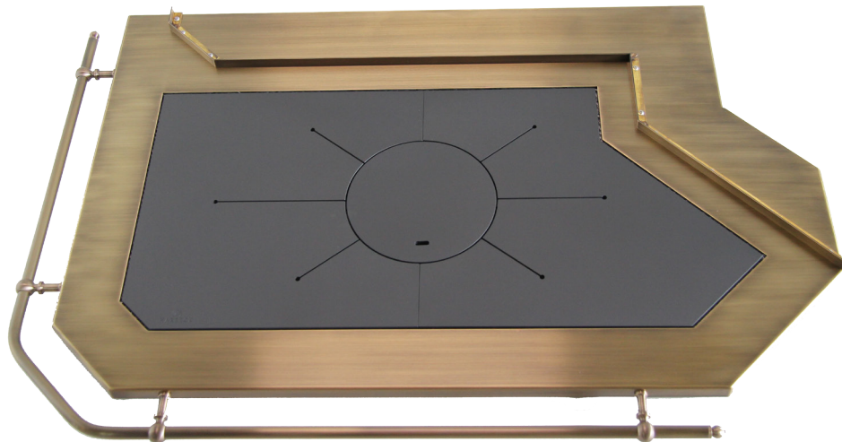
Abb.: Herdrahmen aus Messing antik, mit Wandanschlagleiste Herdplatte aus Hitze-Stahl einbrenngraphitiert geschwärzt
